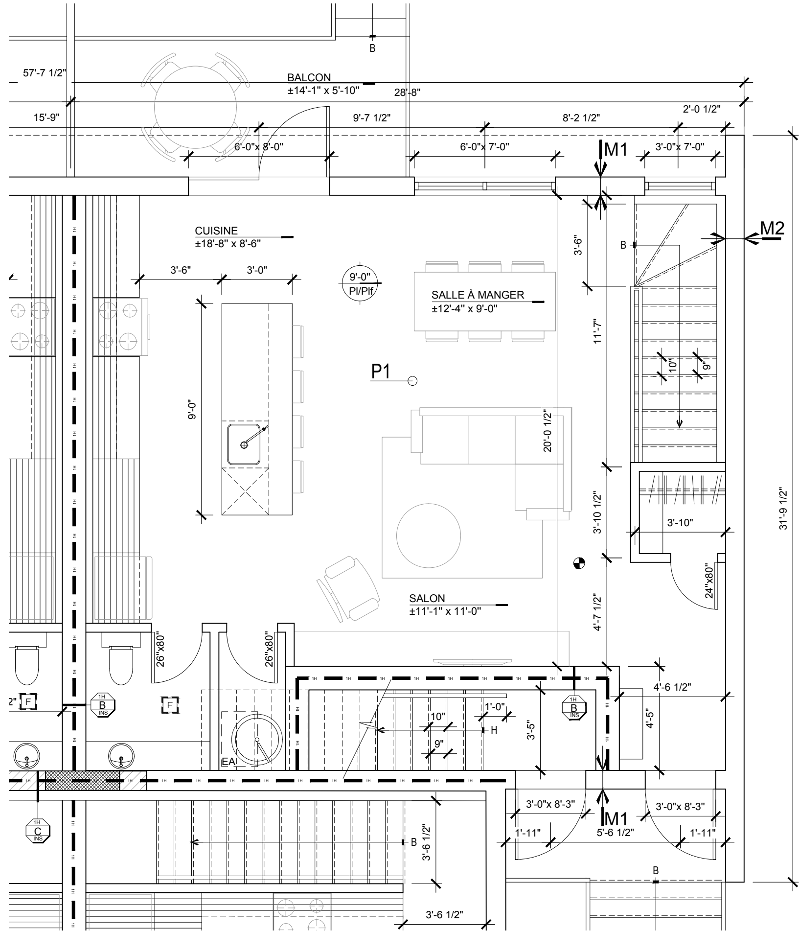
REZ-DE-CHAUSSÉE
