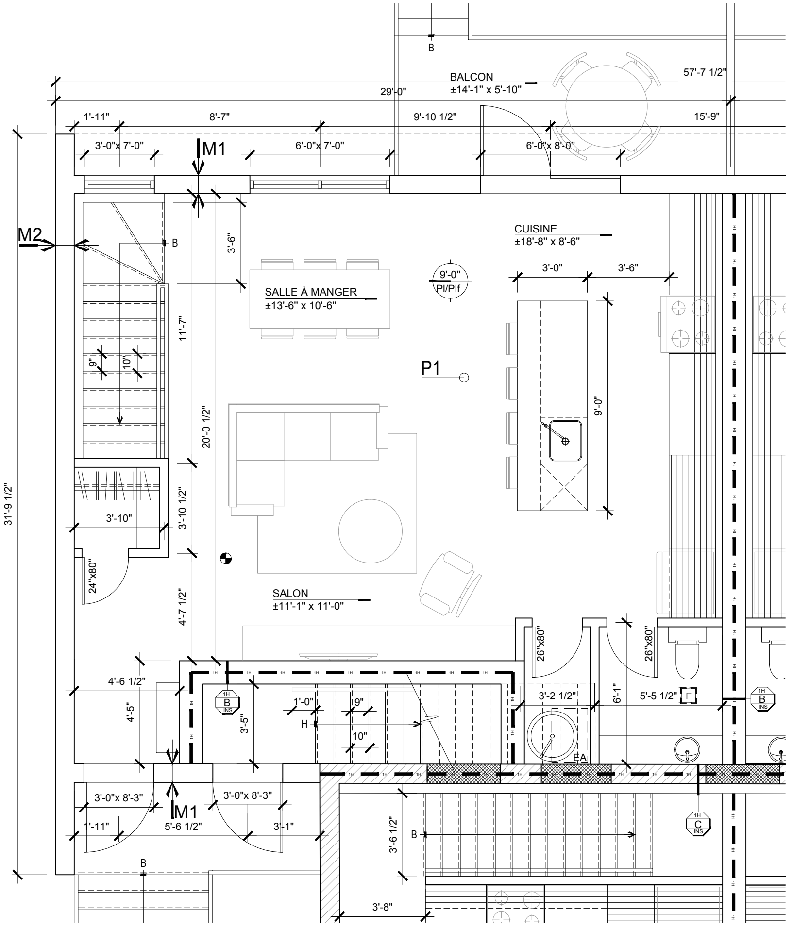
REZ-DE-CHAUSSÉE
