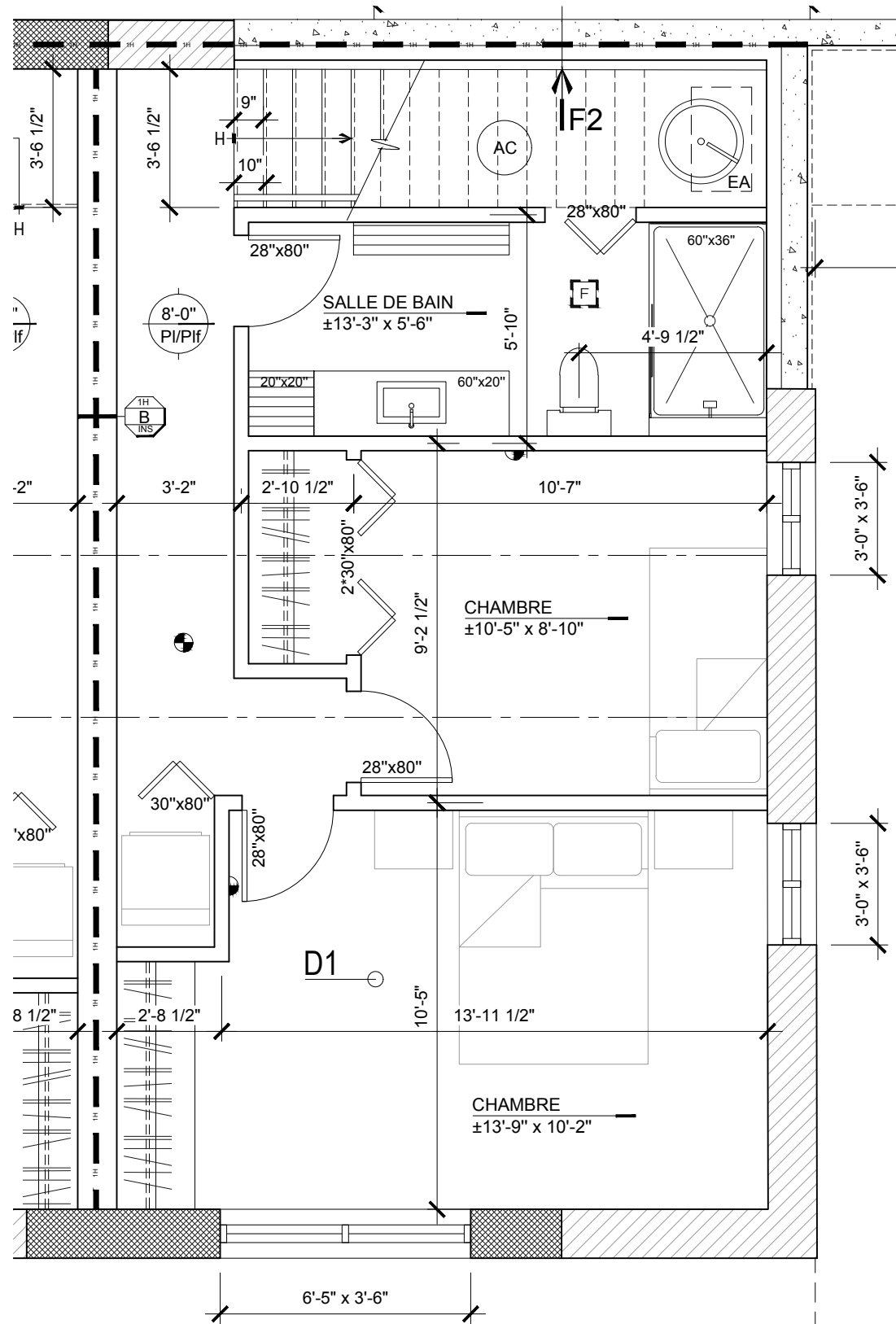
SOUS-SOL
