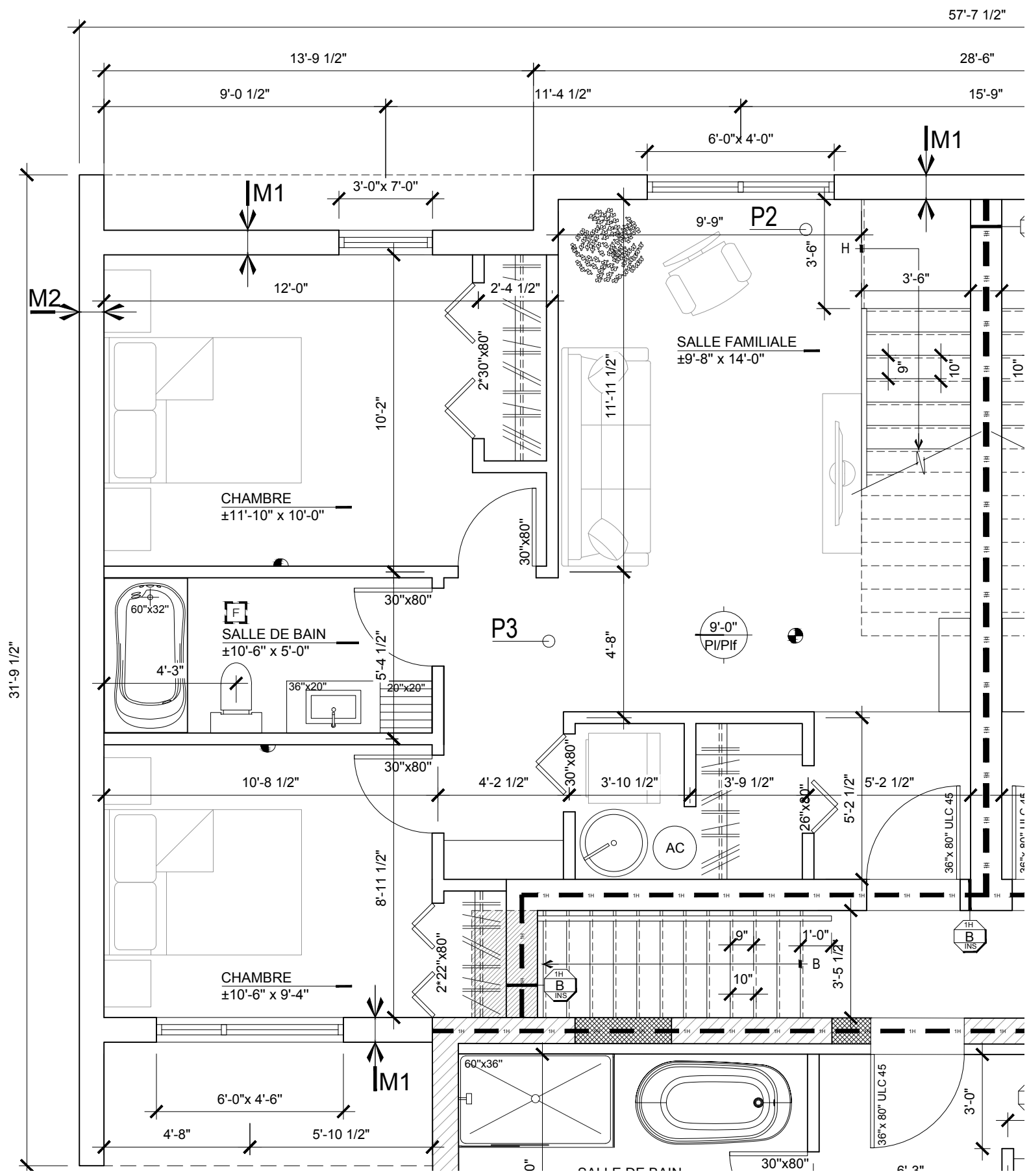
1er ÉTAGE
