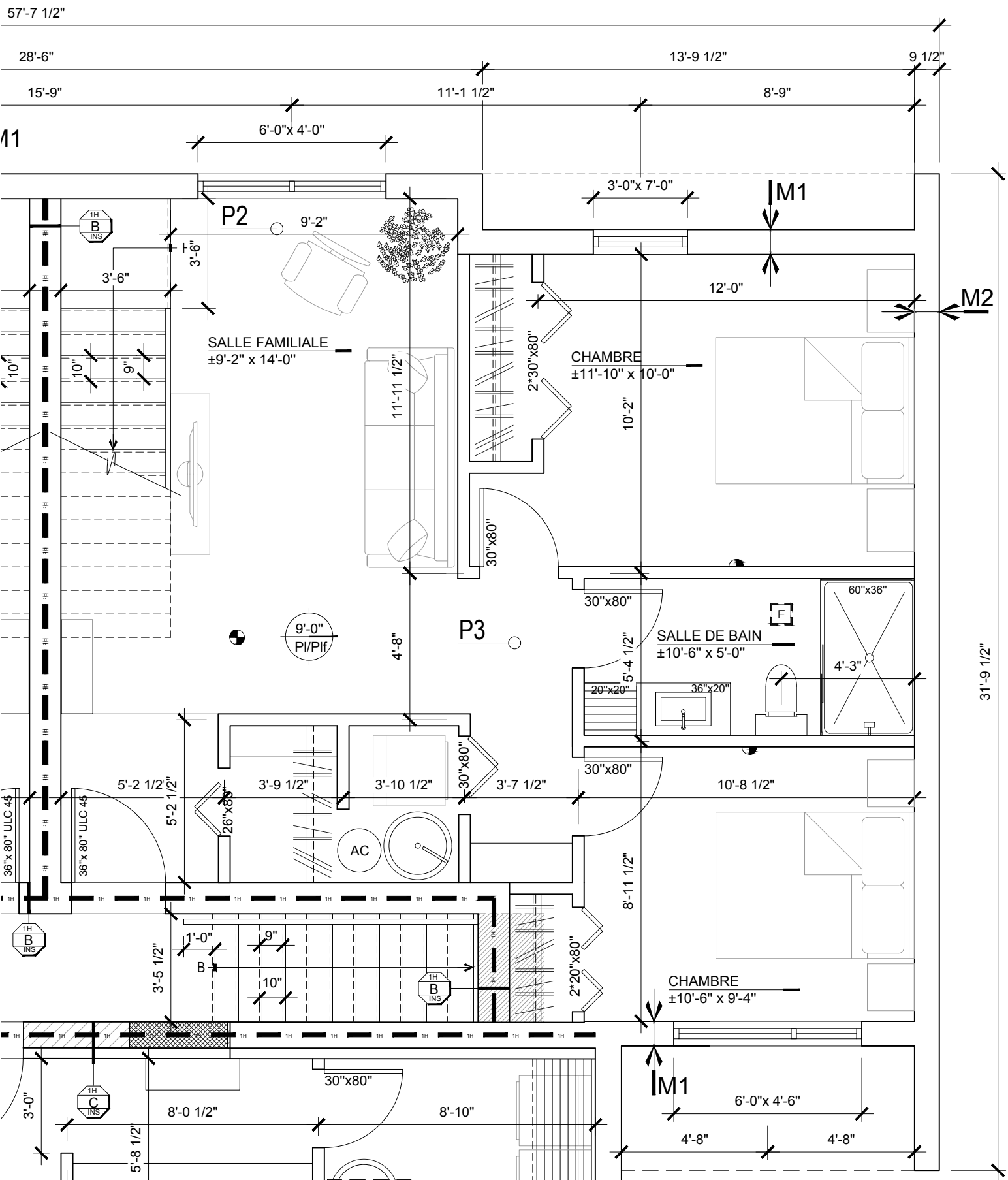
1er ÉTAGE
