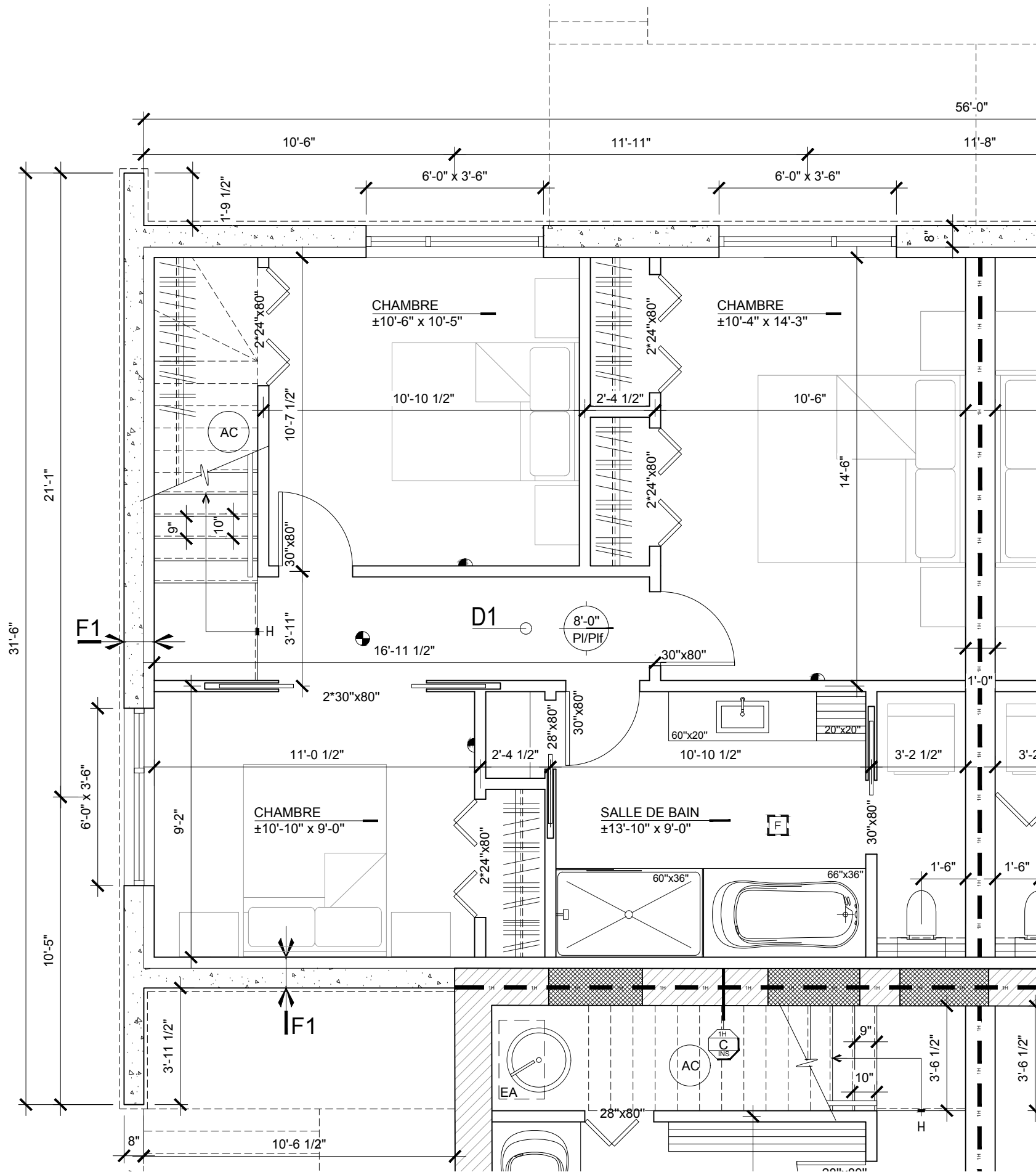
SOUS-SOL
