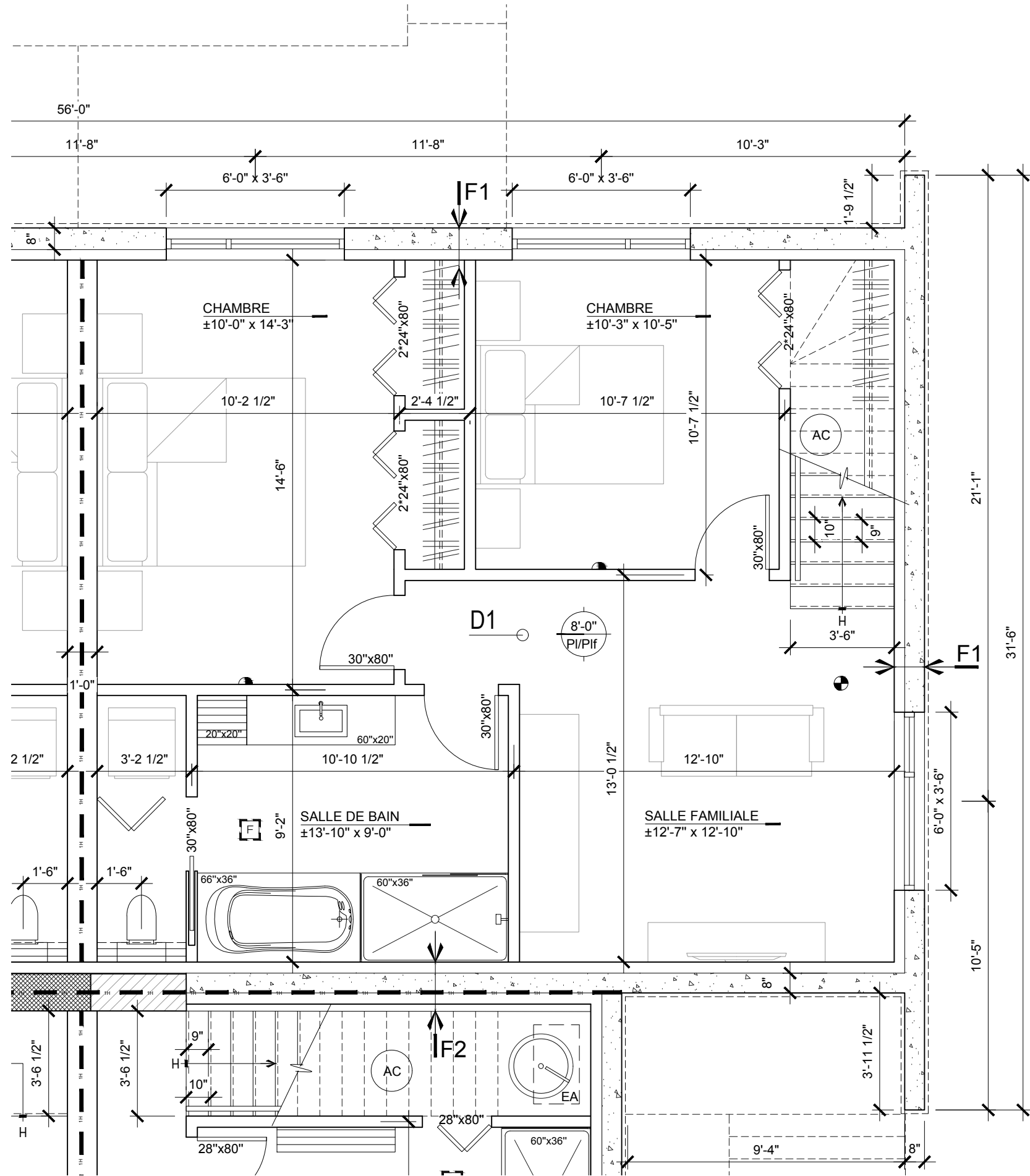
SOUS-SOL
