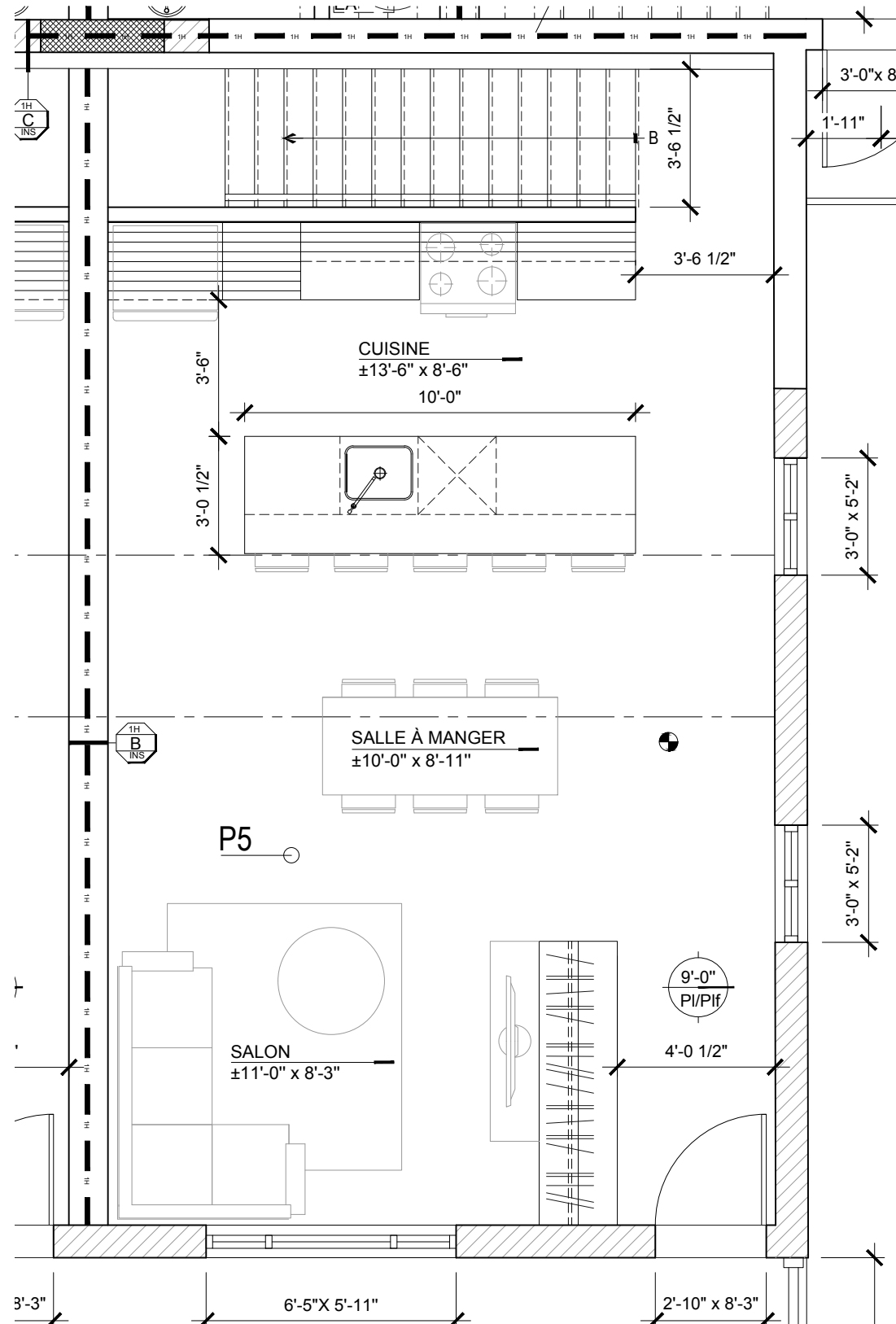
REZ-DE-CHAUSSÉE
