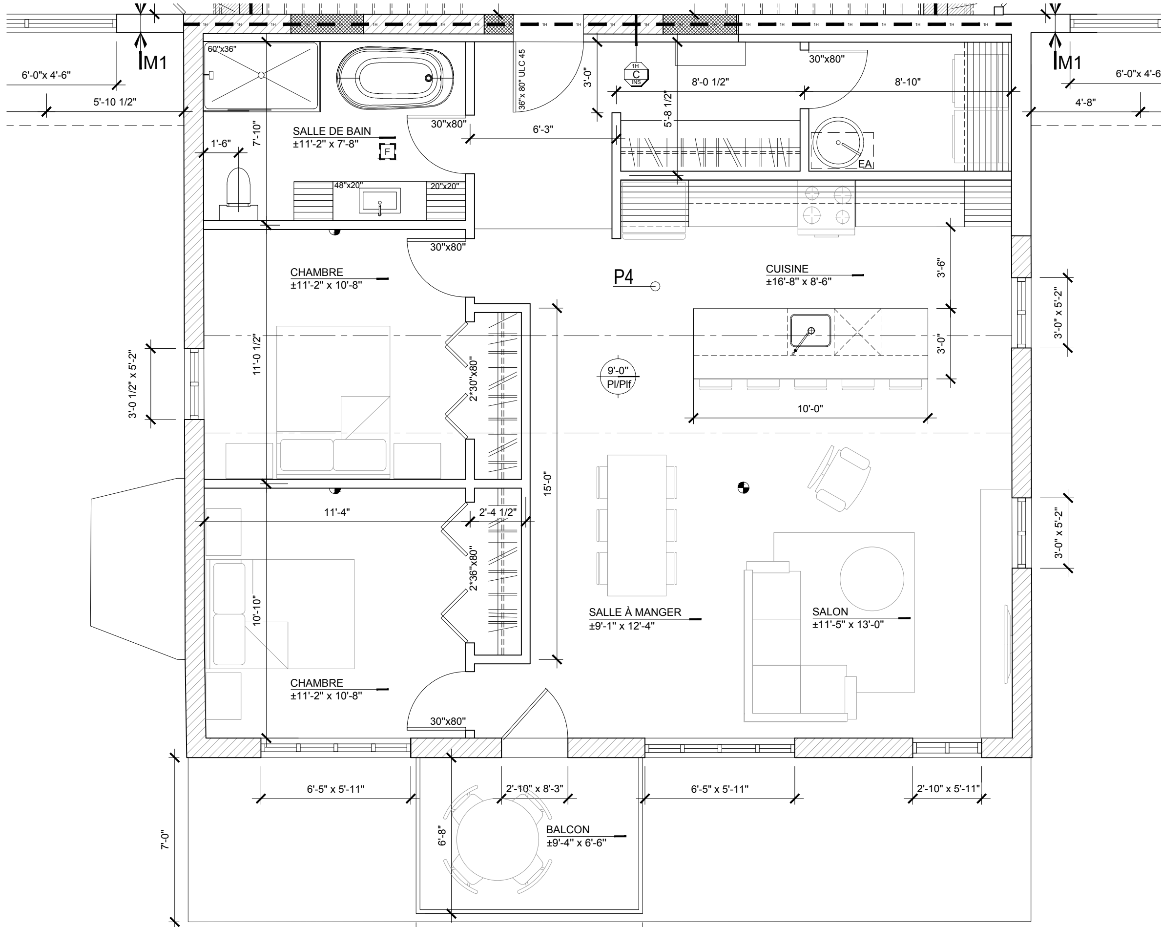
1er ÉTAGE
